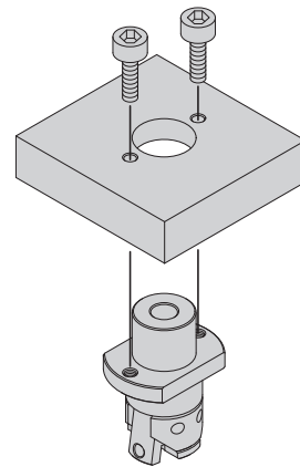
法蘭式固定方式
