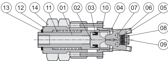
3/4:螺牙後座型(平行/垂直)
